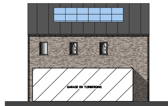
RECHTER ZIJGEVEL
