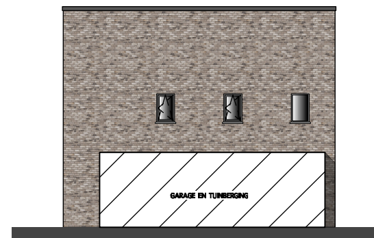
LINKER ZIJGEVEL
