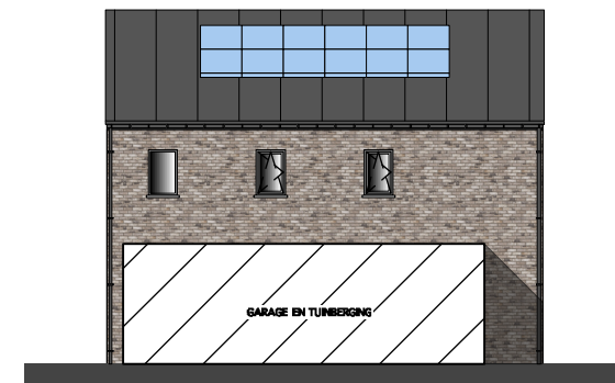
RECHTER ZIJGEVEL
