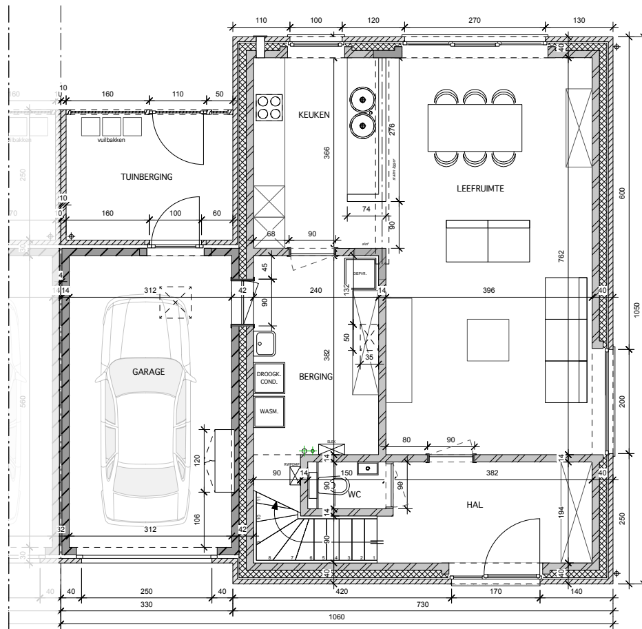
GRONDPLAN GELIJKVLOERS
