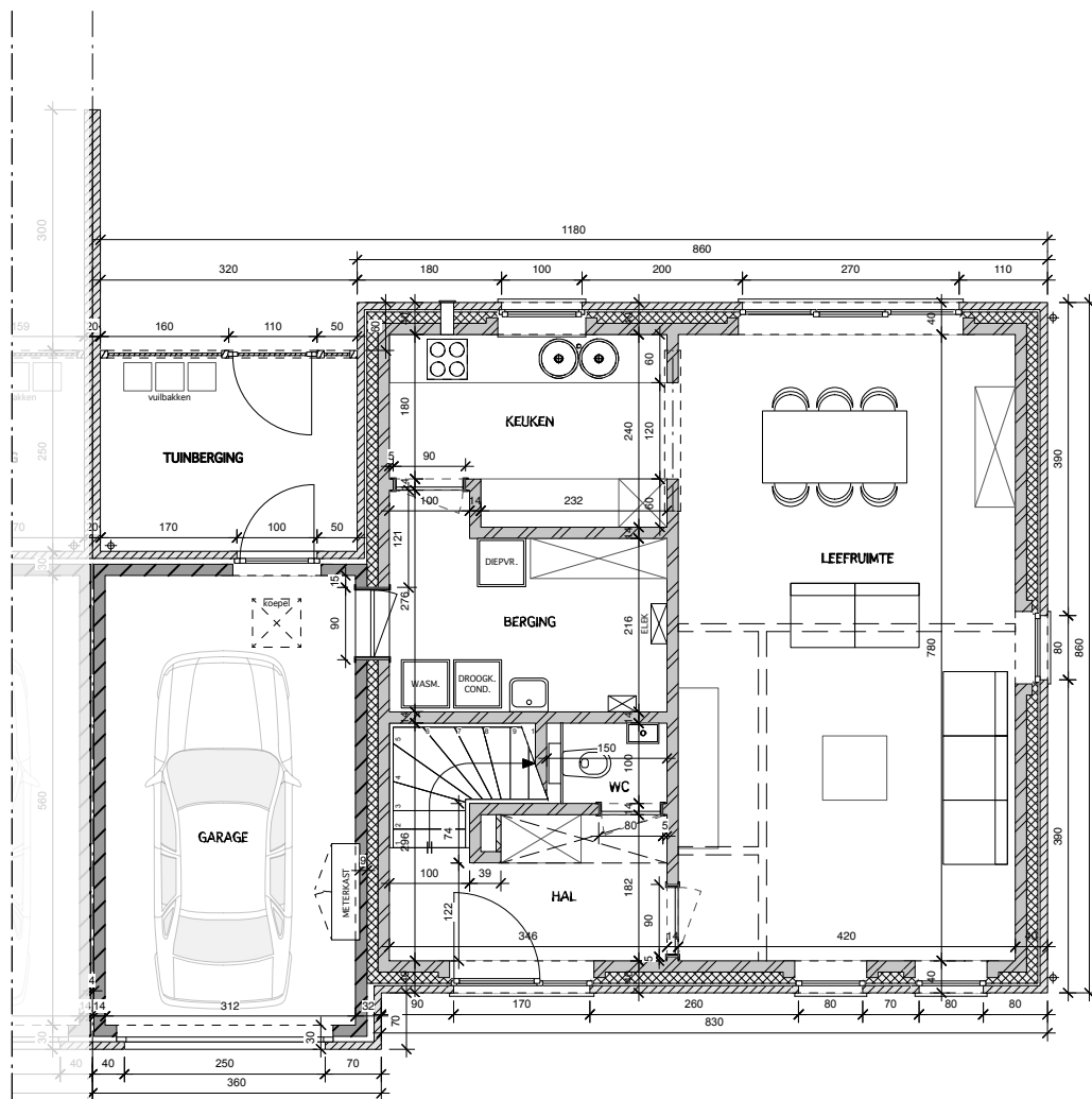
GRONDPLAN GELIJKVLOERS
