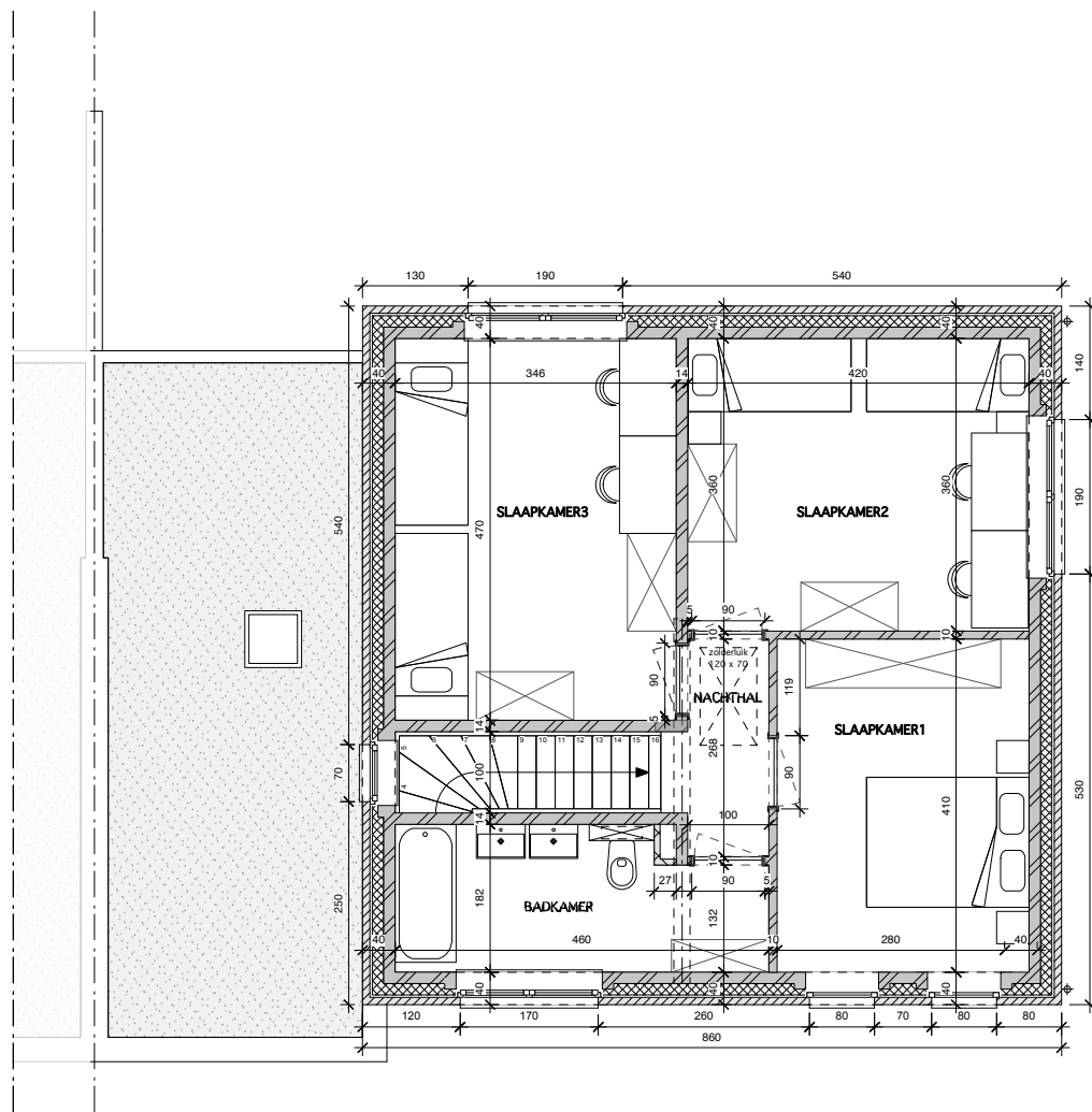
GRONDPLAN VERDIEPING
