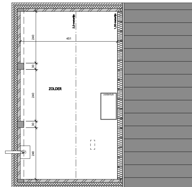
GRONDPLAN ZOLDER
