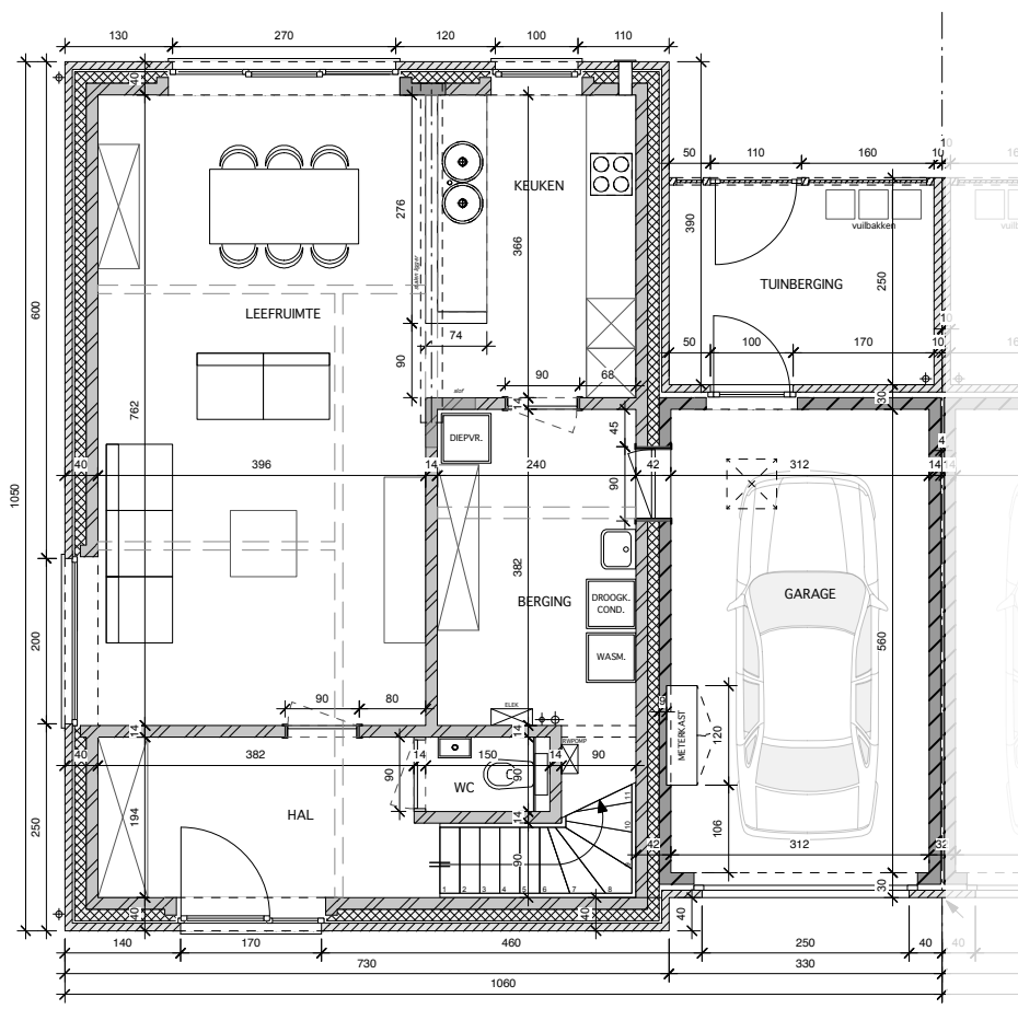
GRONDPLAN GELIJKVLOERS
