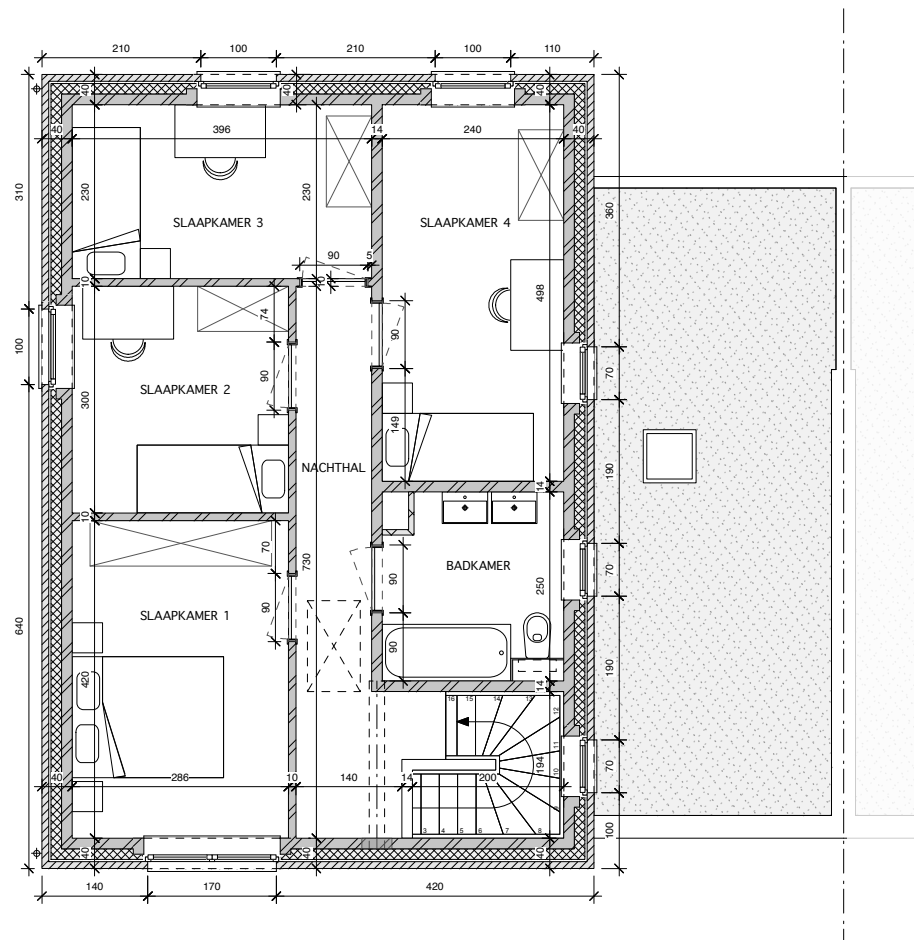
GRONDPLAN VERDIEPING
