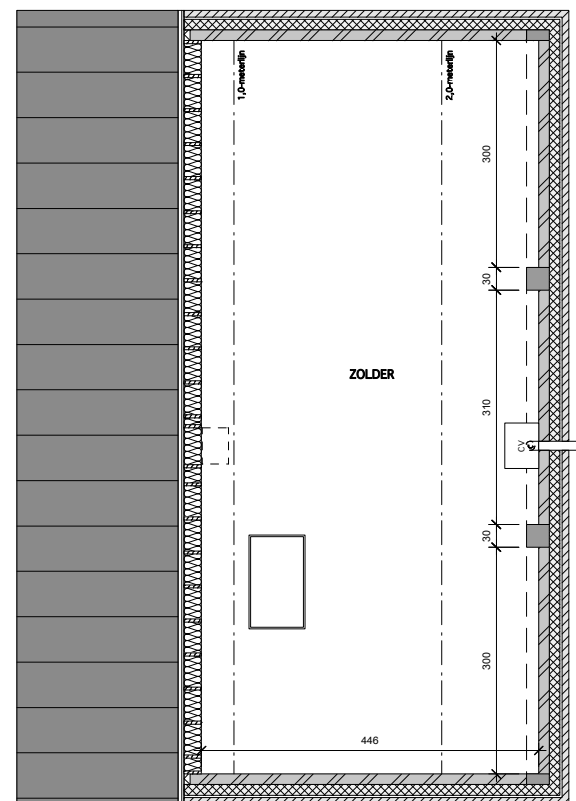
GRONDPLAN ZOLDER
