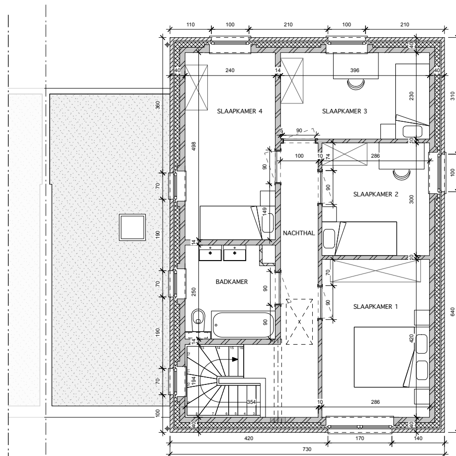
GRONDPLAN VERDIEPING
