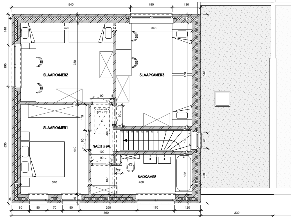
GRONDPLAN VERDIEPING
