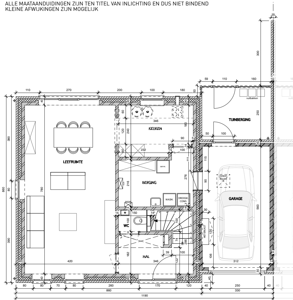
GRONDPLAN GELIJKVLOERS
