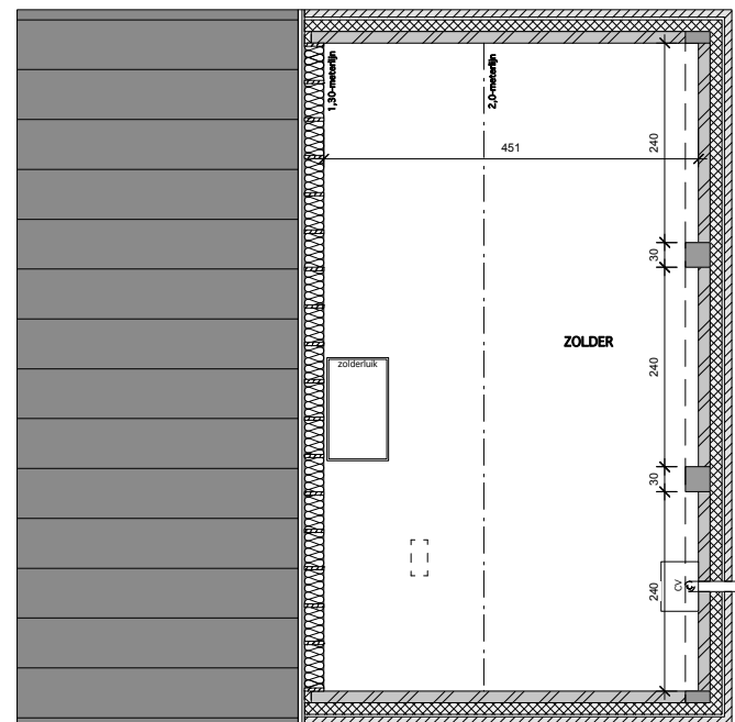
GRONDPLAN ZOLDER
