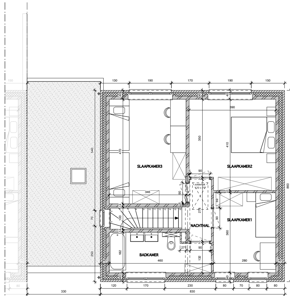
GRONDPLAN VERDIEPING
