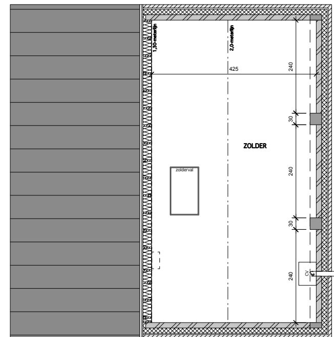
GRONDPLAN VERDIEPING
