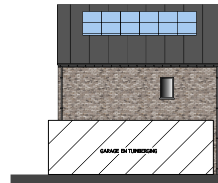
LINKER ZIJGEVEL
