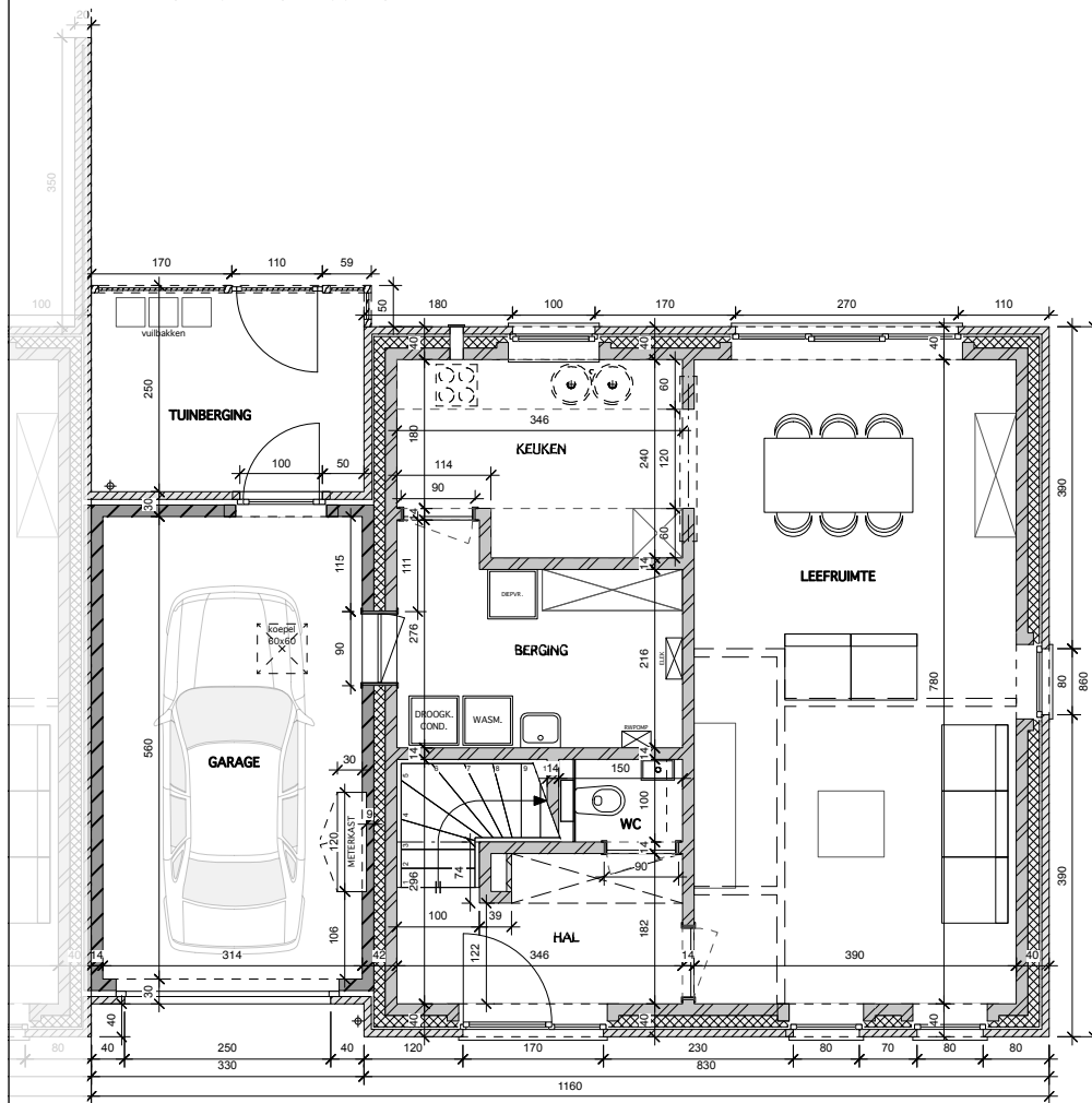
GRONDPLAN GELIJKVLOERS
