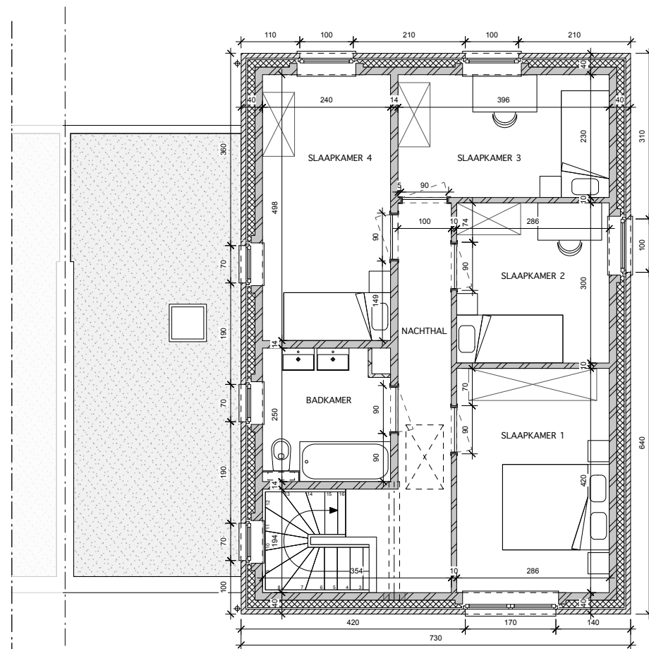
GRONDPLAN VERDIEPING
