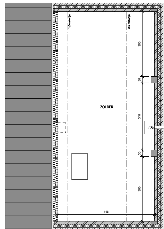
GRONDPLAN ZOLDER
