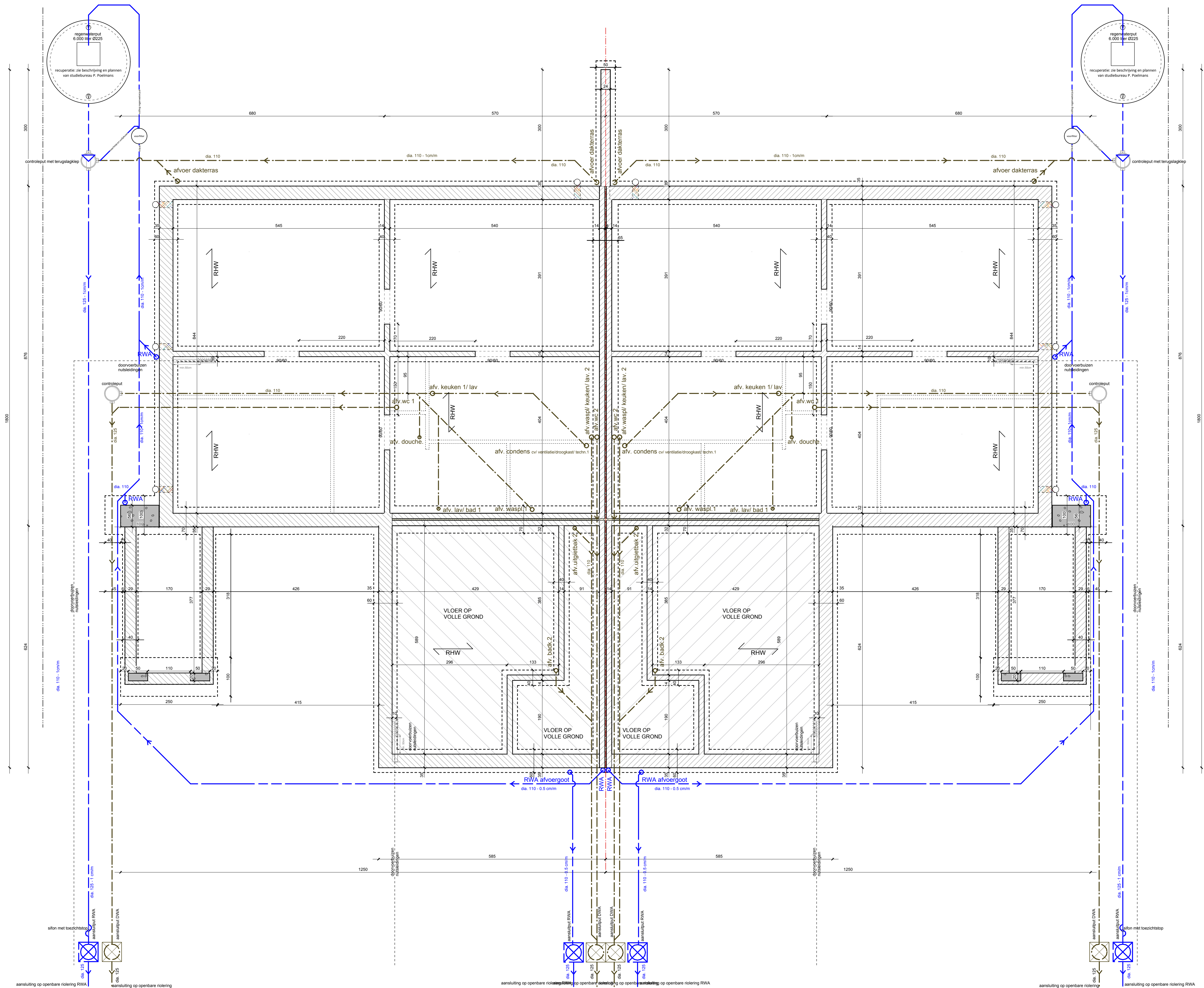
Funderings- en rioleringsplan-schaal 1/50
