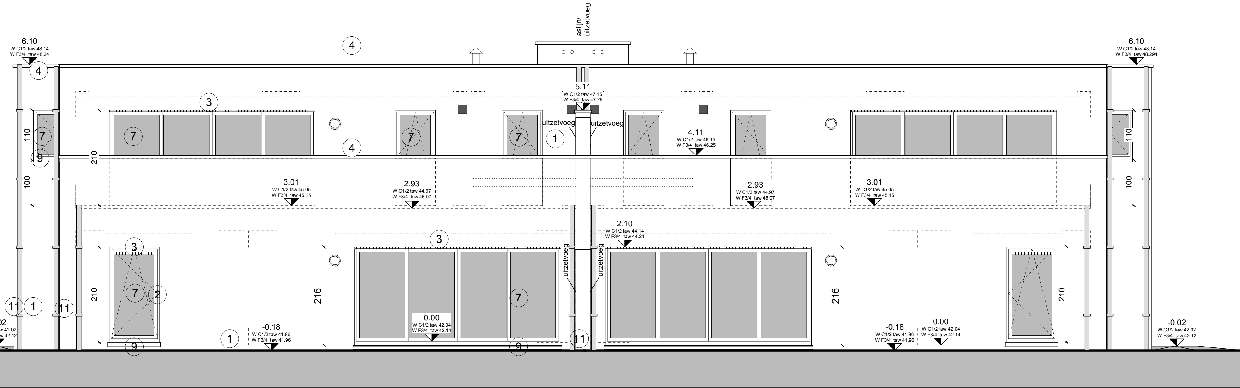
Achtergevel-schaal 1/50
