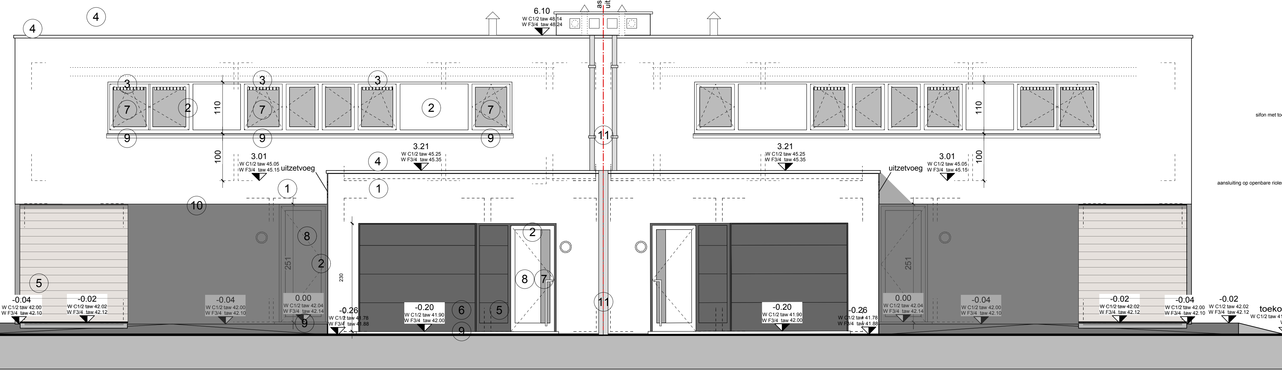
Voorgevel-schaal 1/50
