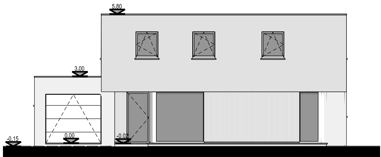
RECHTERGEVEL
